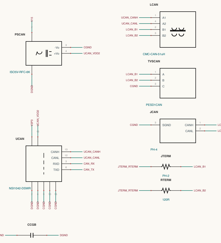
LLC-LESS / BUS-R
